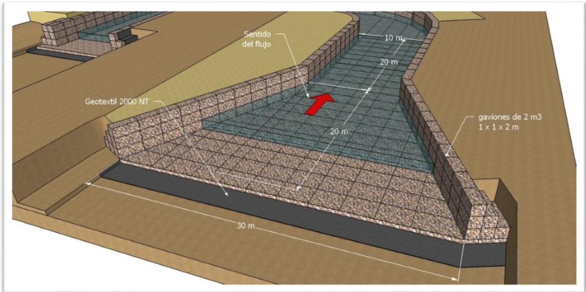
Figura 3: Perspectiva del encole
