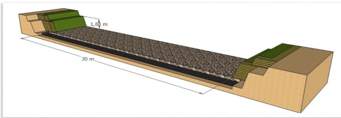
Figura 7: Sección C-C'
