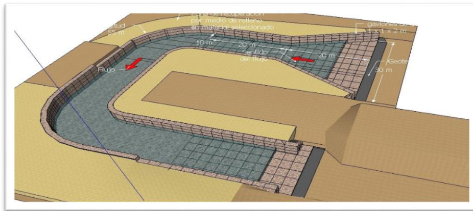
Figura 2: Encole de sistema
