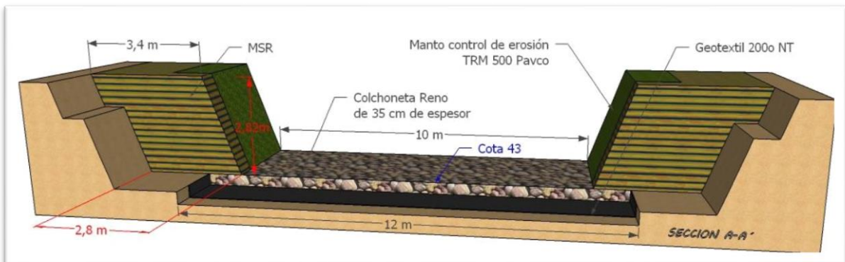
Figura 4: Detalle sección A-A'
