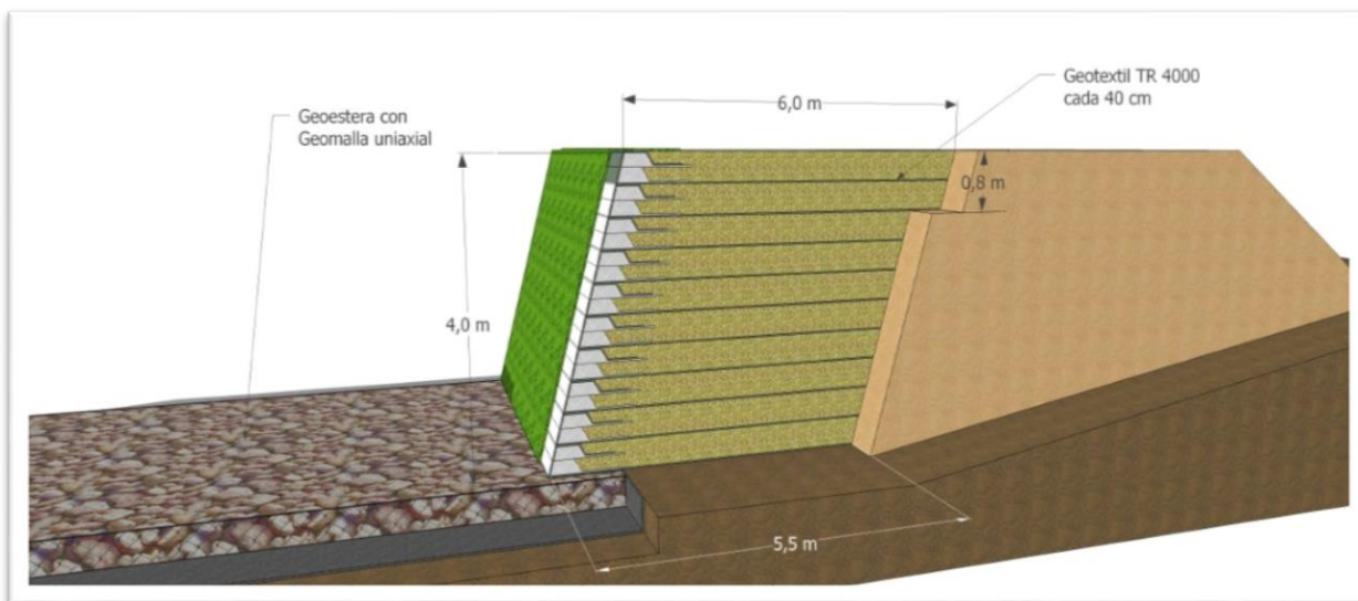
Figura 9.: Detalle MSR de altura 4 m, base de 5,5 y ancho superior de 6 m
